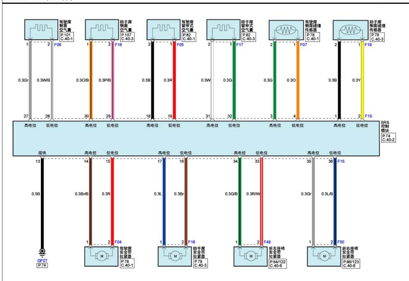
辅助保护系统(SRS)(2)
